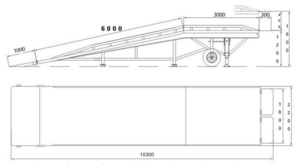
B-TYPE (상부 3.0m) · 외형 도면
